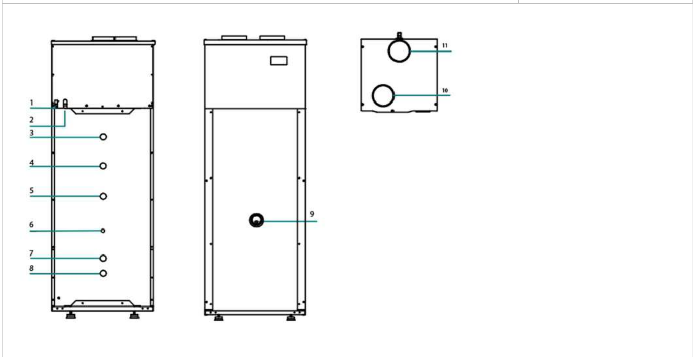
Figura 4. Conexiones traseras
