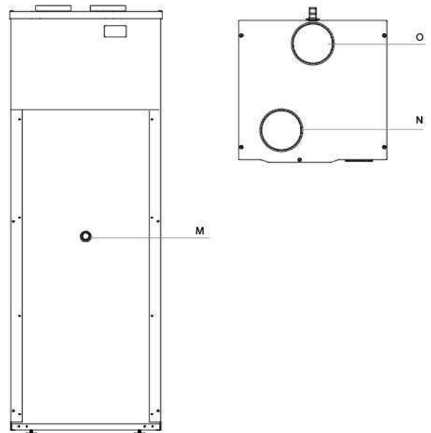
Figura 5. Conexiones delanteras
