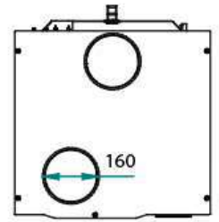
Figura 3. Dimensiones, mm
